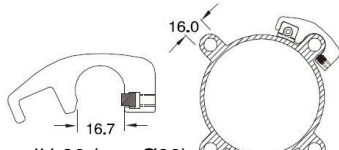
УН-80 (для Ø80)
