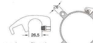
ИН-200 (для Ø200)
