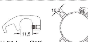
УН-50 (для Ø50)
