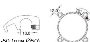
ИН-50 (для Ø50)
