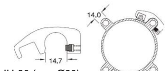
ИН-80 (для Ø80)
