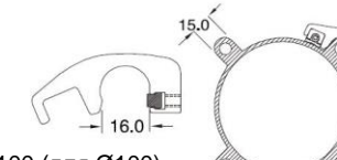
ИН-100 (для Ø100)
