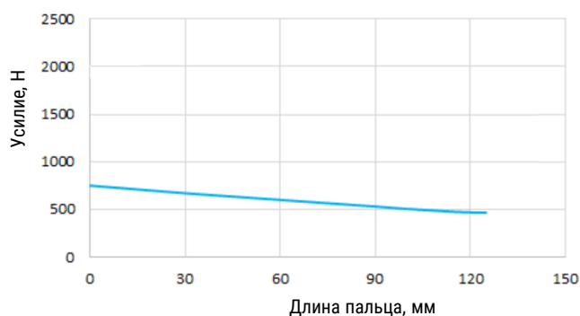
Зависимость усилия открытия от длина пальца
