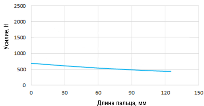
Зависимость усилия закрытия от длина пальца
