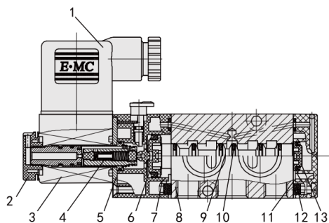
Моностабильный распределитель
