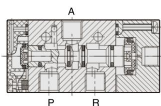
Моностабильный распределитель НО
